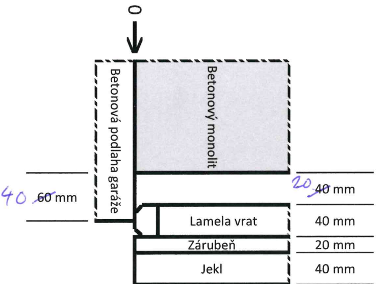
Řez ukončení podlahy
