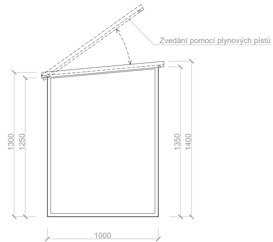
Boční pohled
