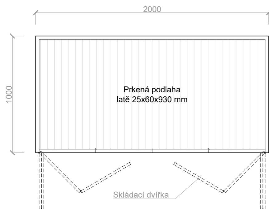
Půdorys
