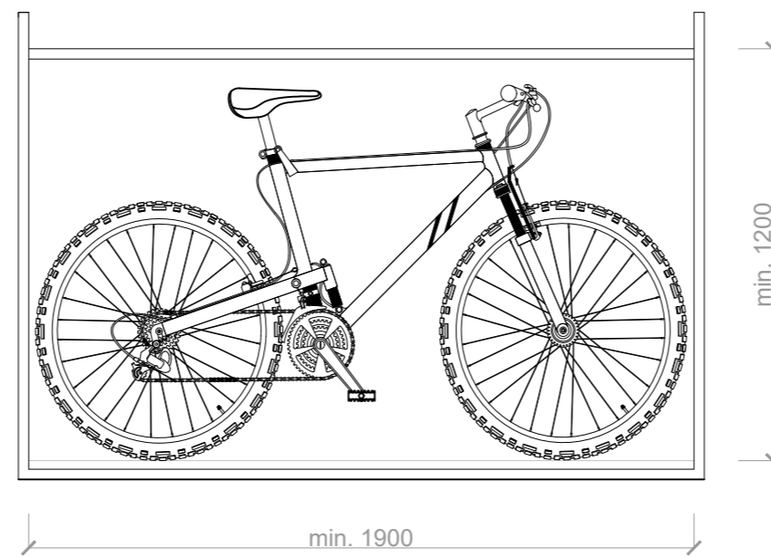
Pohled uložení kola
