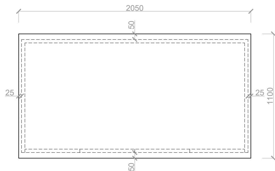
Půdorys
