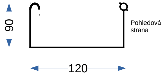
Řez stávajícím žlabem
