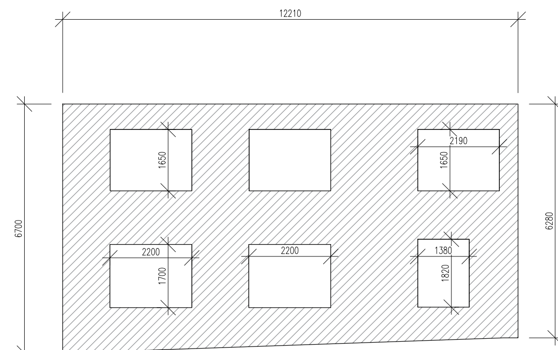
POHLED VÝCHODNÍ
