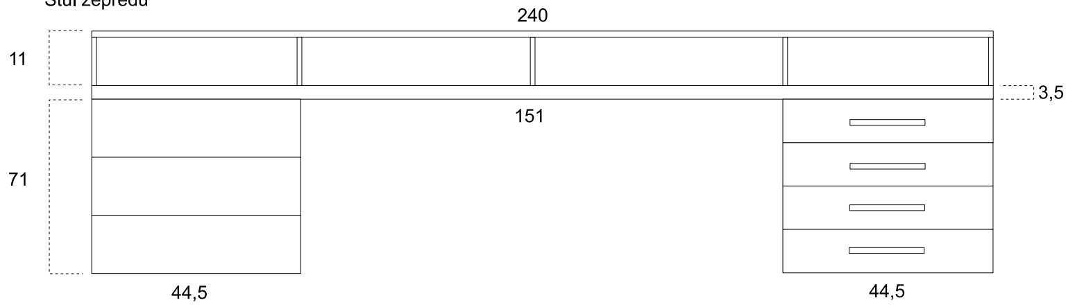
Stůl zepředu
